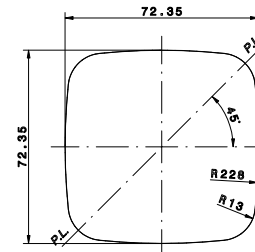
Section cut B-B Scale: 1:1
