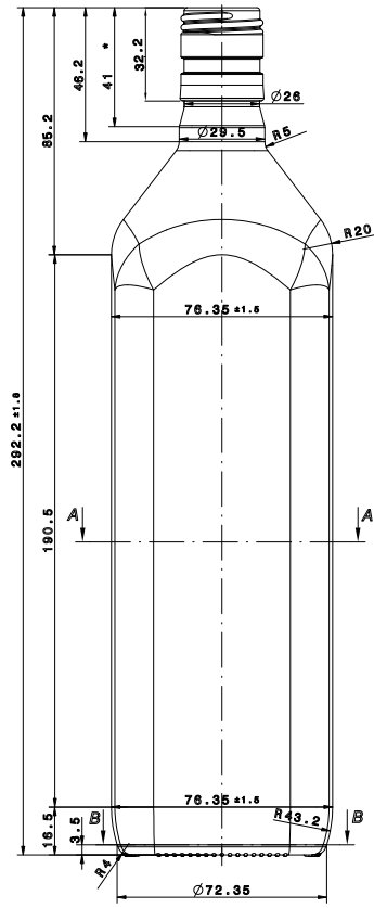
Front view Scale: 1:1
