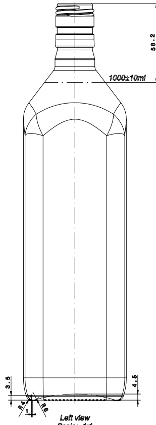
Left view Scale: 1:1
