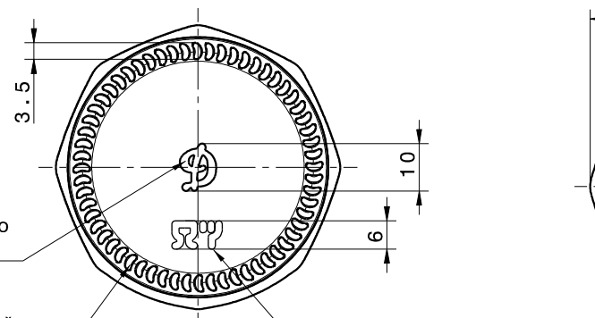
Bottom view Scale: 1:1
