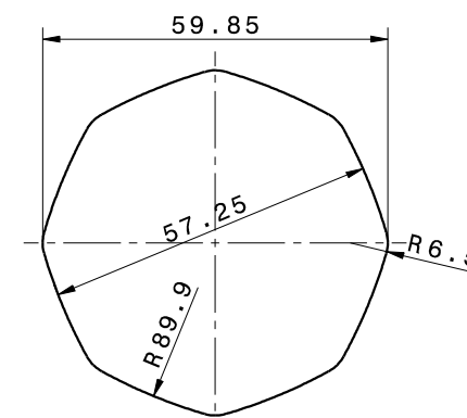
Section cut D-D Scale: 1:1
