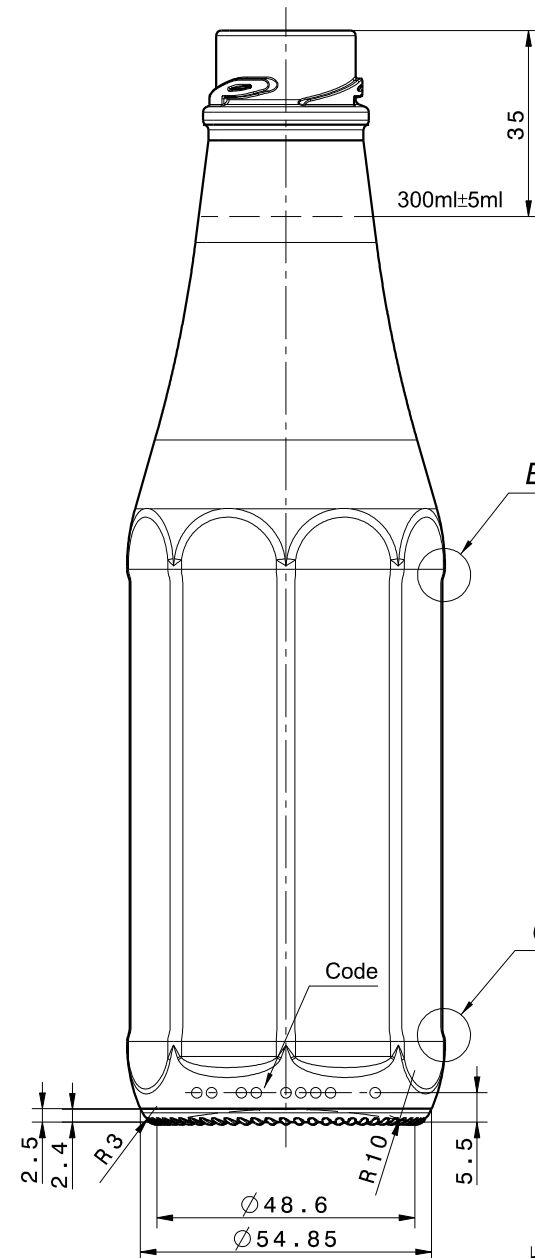
Rear view Scale: 1:1
