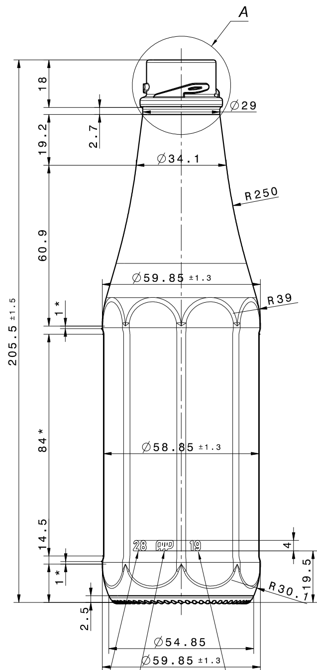
Front view Scale: 1:1
