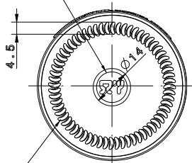
Bottom view Scale: 1:1
