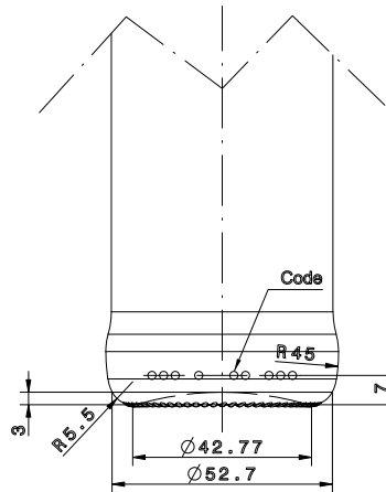
Rear view Scale: 1:1
