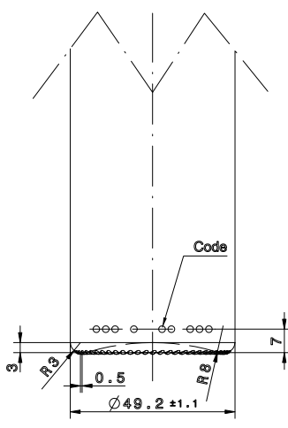
Rear view Scale: 1:1
