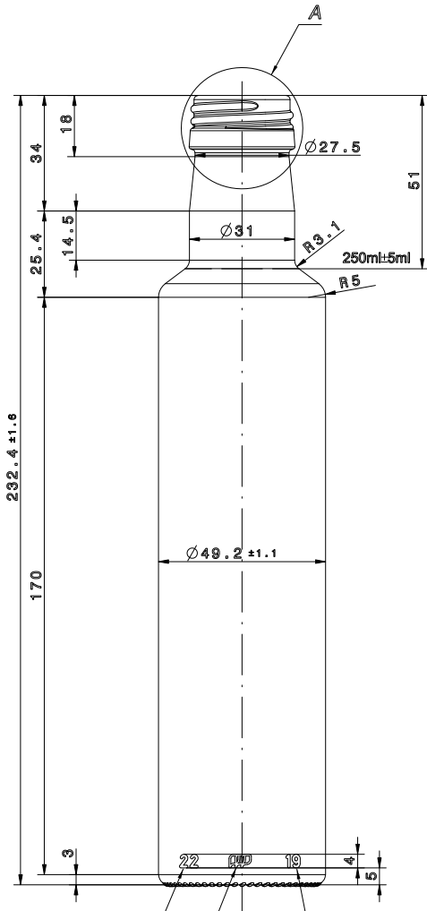
Front view Scale: 1:1
