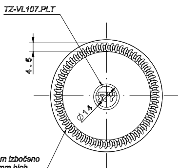
Bottom view Scale: 1:1
