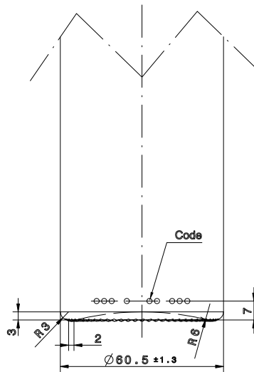
Rear view Scale: 1:1
