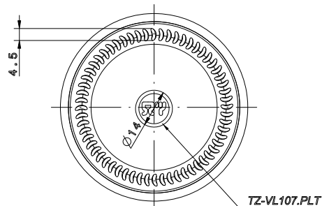
Bottom view Scale: 1:1
