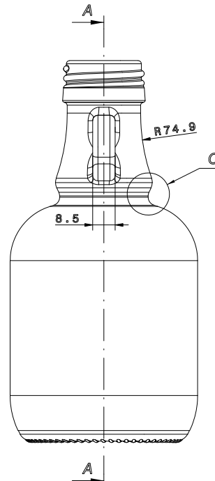
Right view Scale: 1:1
