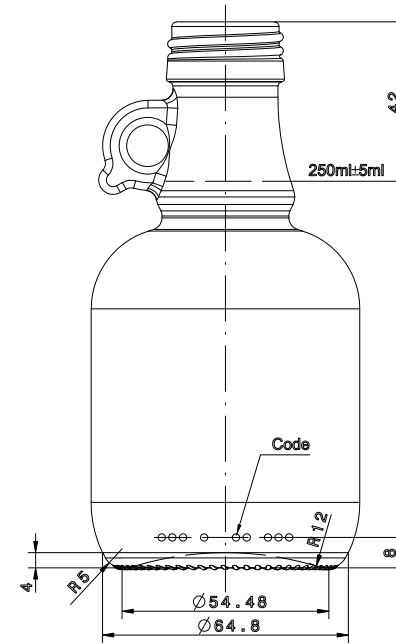
Rear view Scale: 1:1
