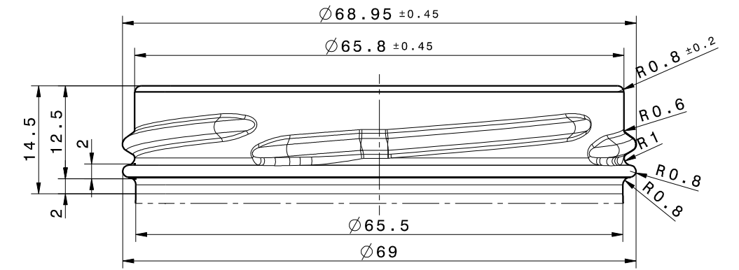
Detalj A M 2:1
