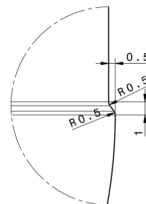
Detalj B M 5:1
