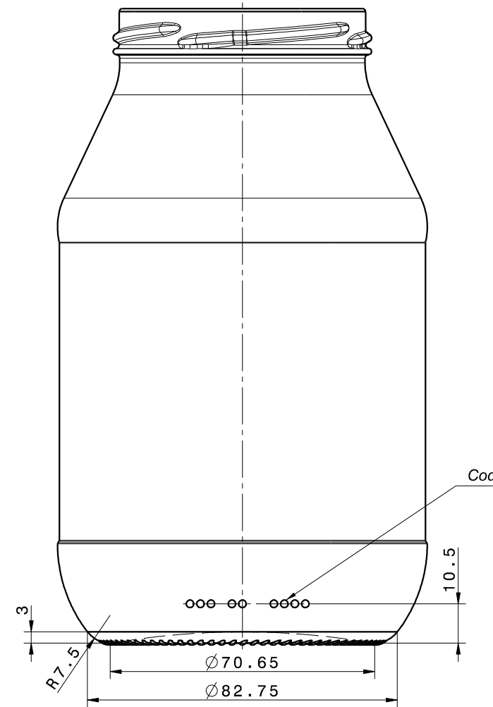
Left view Scale: 1:1
