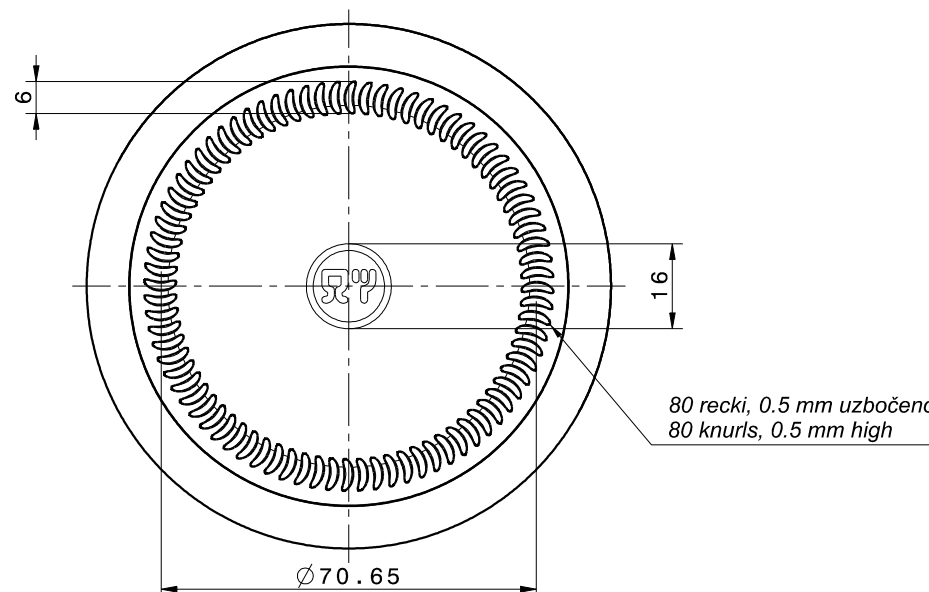
Bottom view Scale: 1:1
