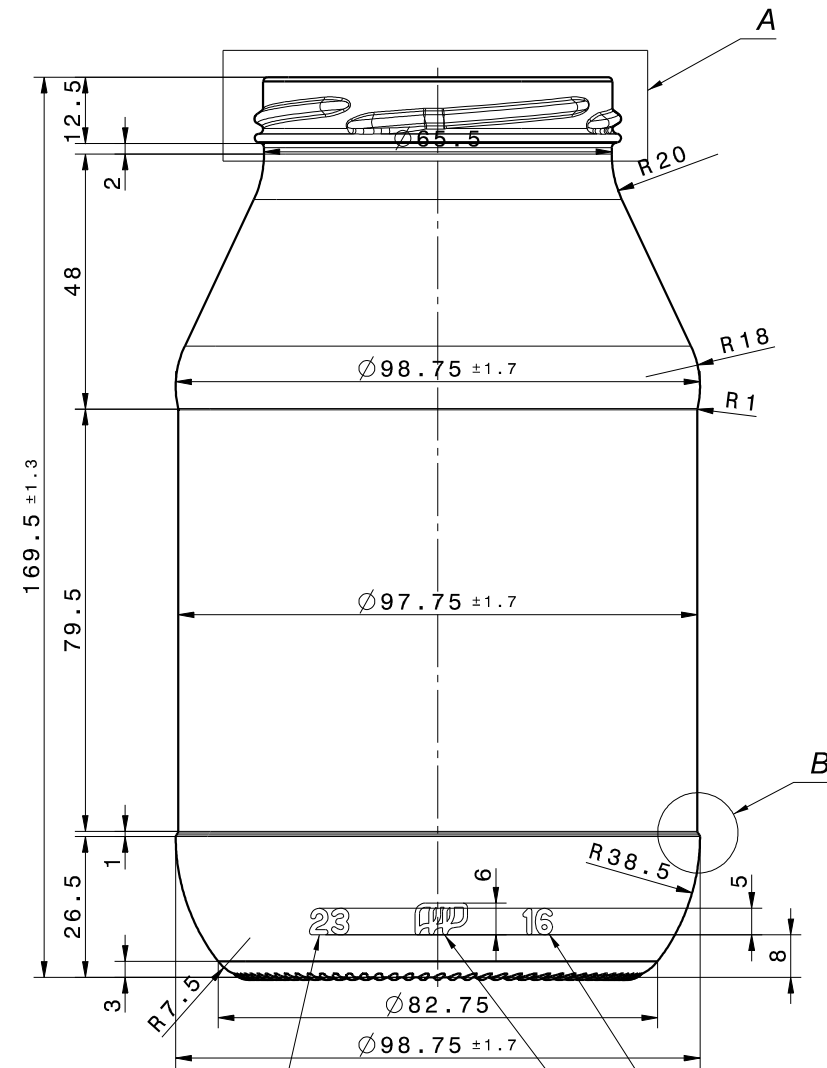
Front view Scale: 1:1
