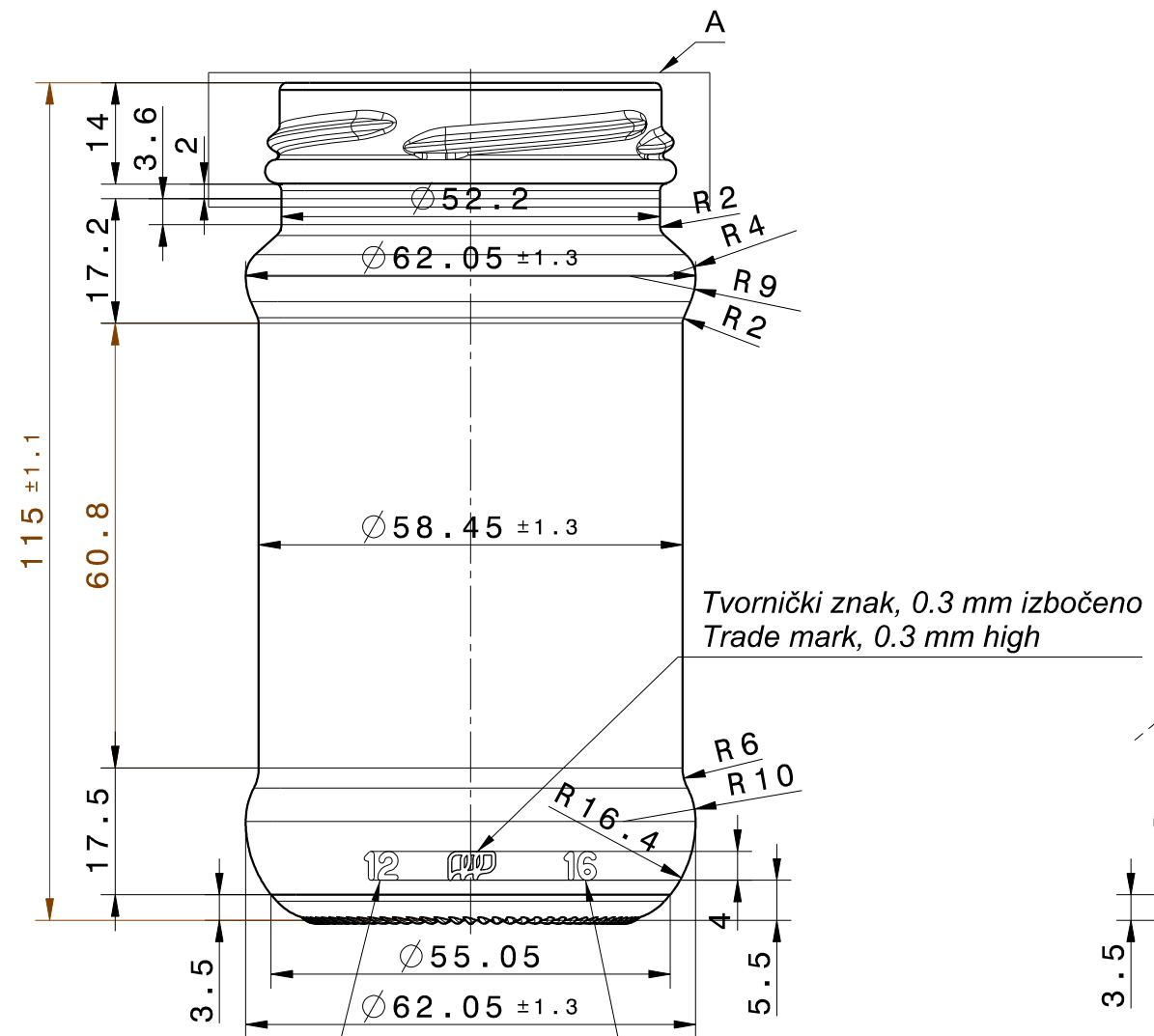
Front view Scale: 1:1
