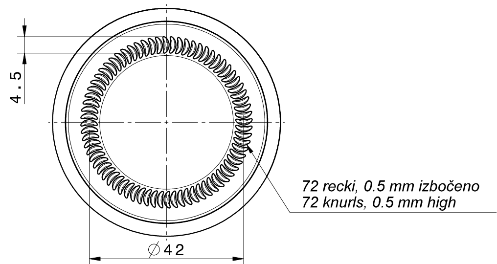
Bottom view Scale: 1:1
